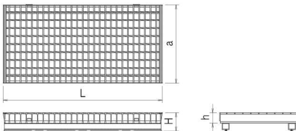
単体図
