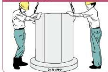
6 受枠高さの微調整とモルタル充填
