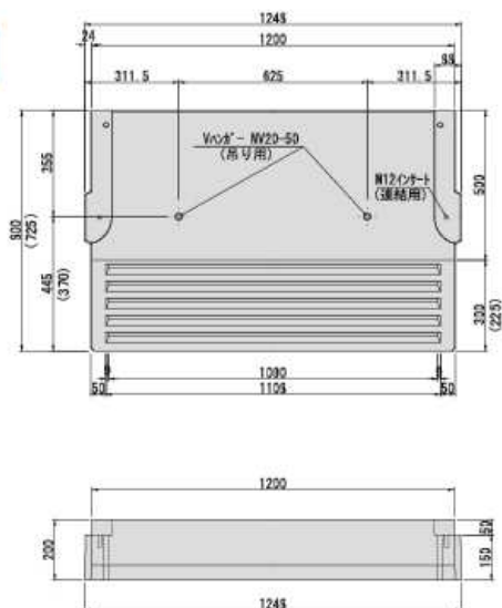
川裏施工断面図
