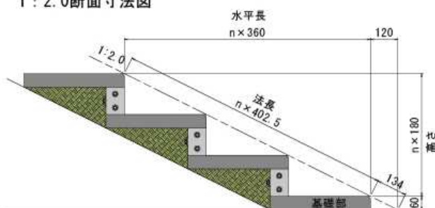
1 : 2.0断面寸法図
