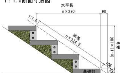
1 : 1.5断面寸法図
