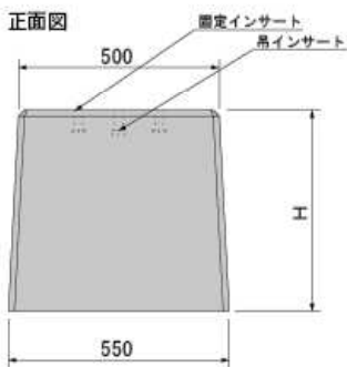
正面図
