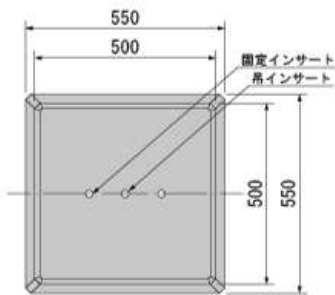
平面図
