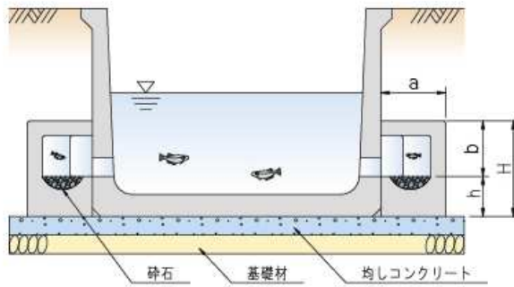
単体図 横断面図
