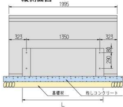
縦側面図
